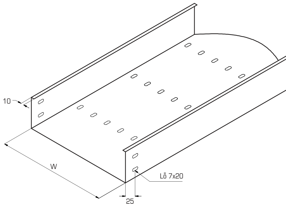
MÁNG THẲNG / STRAIGHT TRAY Mã đặt hàng / Order code: STH-WxHxT
