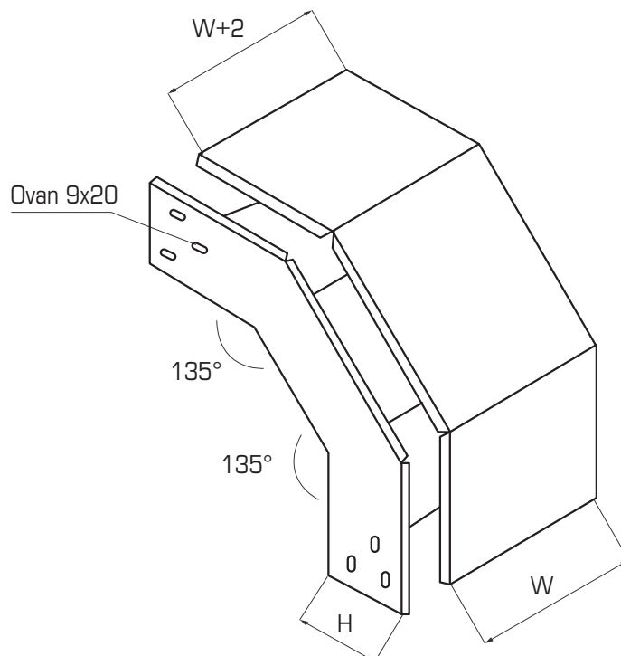
CO XUỐNG / VERTICAL BEND (DOWN) Mã đặt hàng / Order code: EBTR-WxHxT
