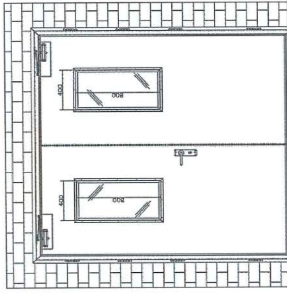
MẶT TRƯỚC
